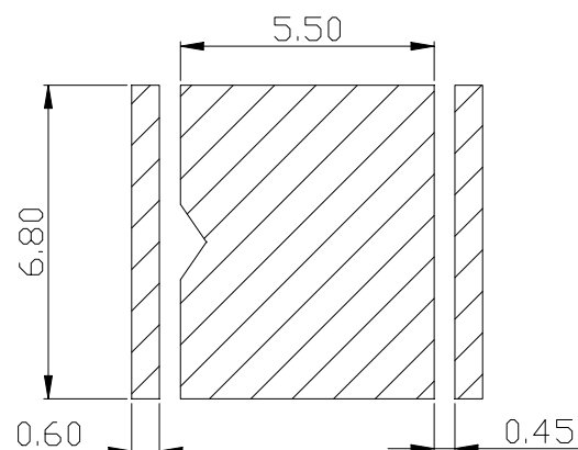
建议焊盘
